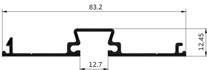
A10261 ดบร่อง 1" (สลิ้ม)
