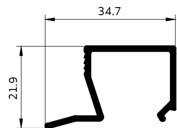
5008 คิ้วกระทุ้ง ช่องแสง UN
