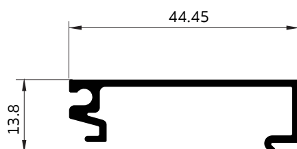
010126 ฝาปิด-เปิด 1"
