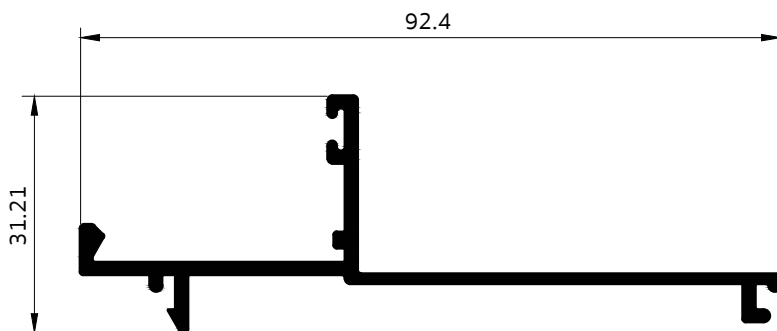
030064 ฟาตบกล่องทึบ กระทุ้ง UN
