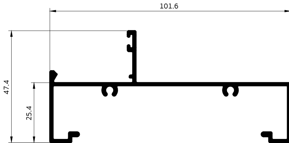
030065 กล่องทึบ 1" กระทุ้ง UN
