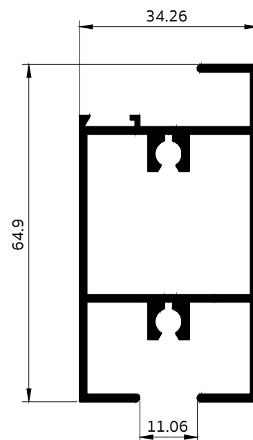
3094 เสาประตูบน-ล่าง บานเปิด 2.5"
