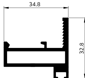
5076 กรอบนอกบานกระทุ้ง
