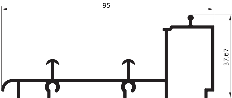
4394 เฟรมล่างขาสูง (ไม่มีจากกันตก)
