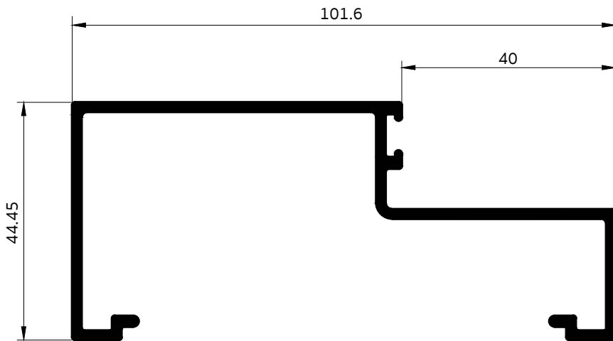
3097 วงกบไม้ 1.75 มม. (ไม่มีตั้ง)
