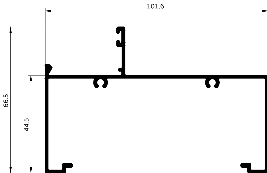
030131 กล่องทึบ 1" 3/4 กระทุ้ง UN
