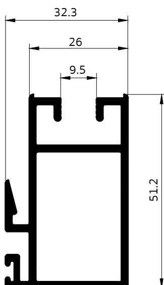
14005 เสาทึบ 2"
