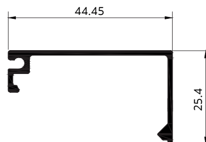
A10258 ฝาปิด-เปิด 1" (สลิ้ม)
