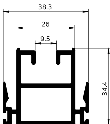
14007 เสาทึบ 2 ทาง
