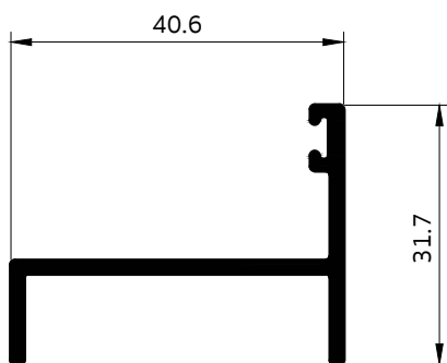
5080 กรอบนอกขาเก้า
